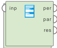
Optimize Parame...
